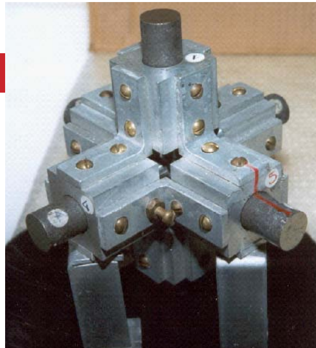
TENSOR DE ESPACIO MAGNÉTICO (TEM) Construido en 1994 por el Ingeniero Ricardo de Godoy Andrade. Con este equipo Andrade pudo crear un Campo Biomagnético (CBM). Este aparato no utiliza energía eléctrica. Está compuesto de seis imanes de alnico (aleación de aluminio, níquel y cobalto)
